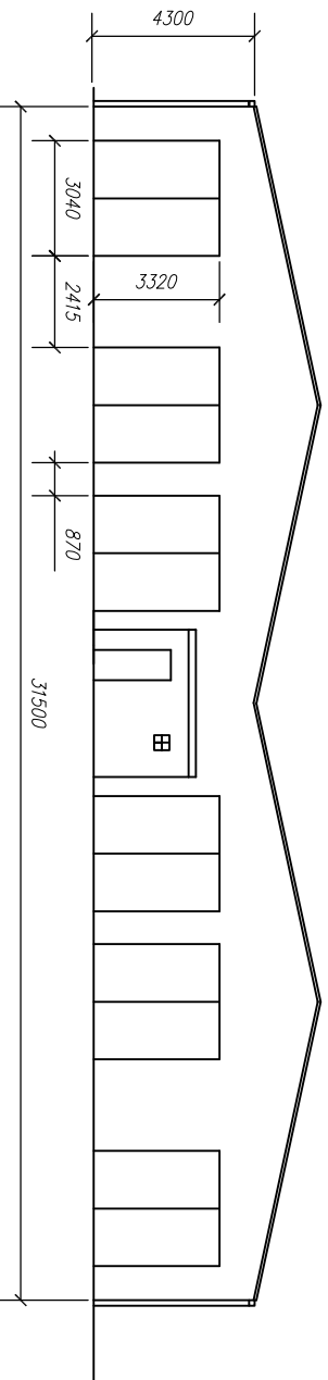
Severní pohled
